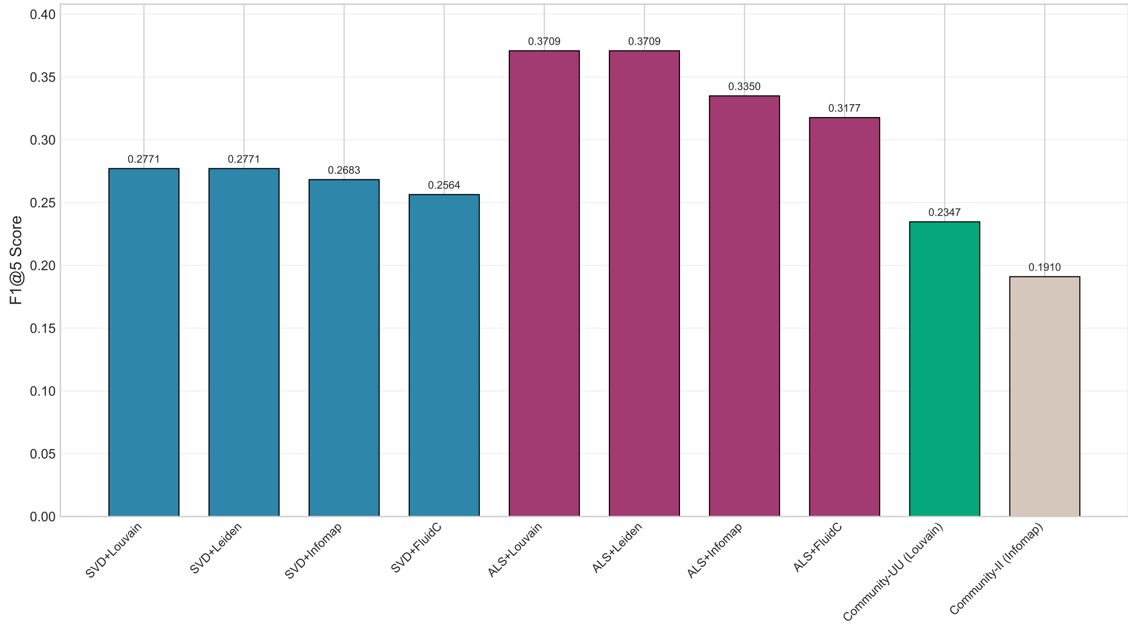
Figure 37: SVD and ALS Hybrids vs. Pure Community Baselines
